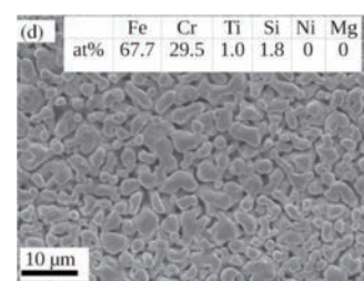
図2 作製したフェライト系ポーラスステンレスのSEM写真と組成分析結果
