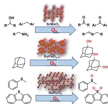
図1 ペロブスカイト触媒による \text{O}_2 のみを用いた選択酸化反応
