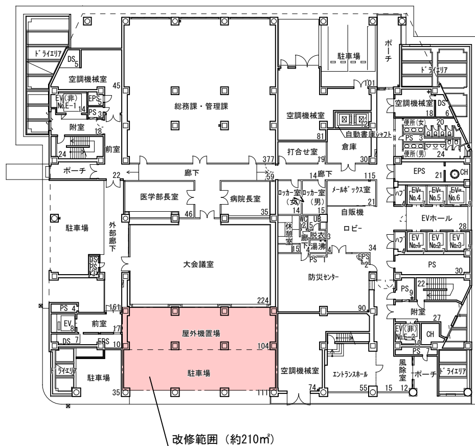
M & Dタワー 1階平面図 (S=1/500)
